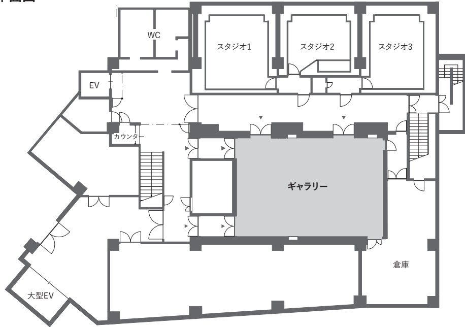
B1 平面図
