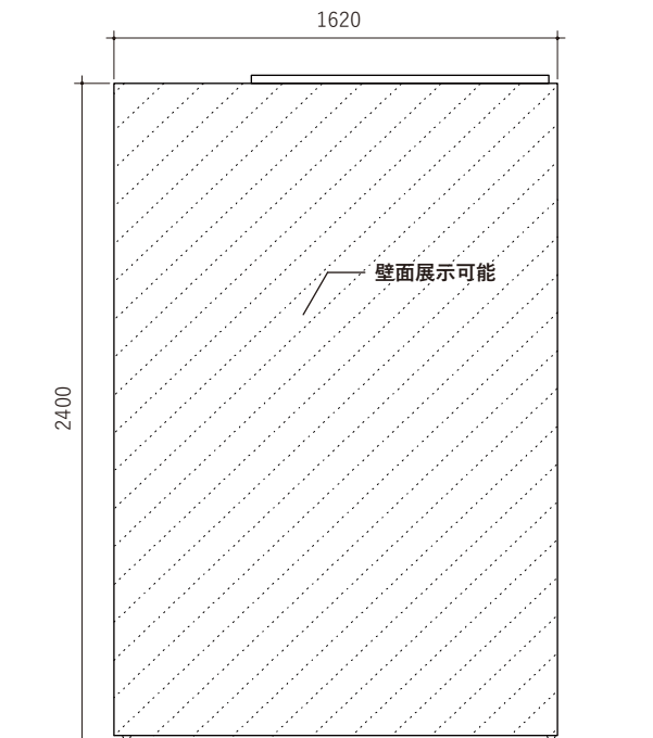
A正面図
