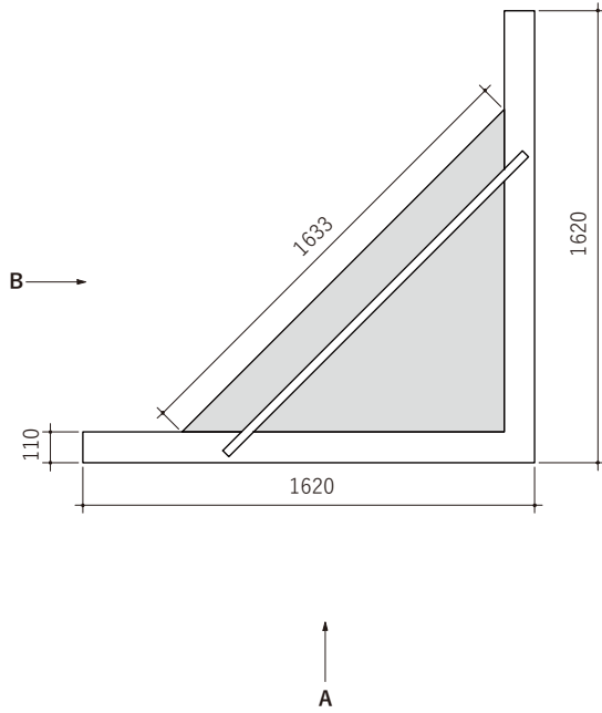
平面図
